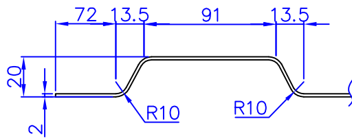
DETAIL C 2:1
