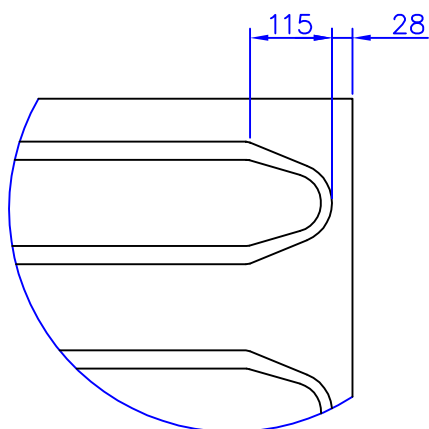
DETAIL B 2:1
