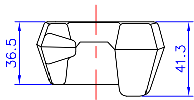
CIMC-D23-02A LH (左)
