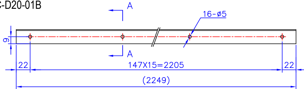
CIMC-D20-01C
