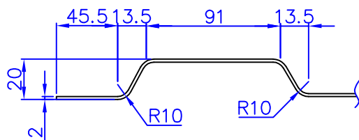
DETAIL C 2:1
