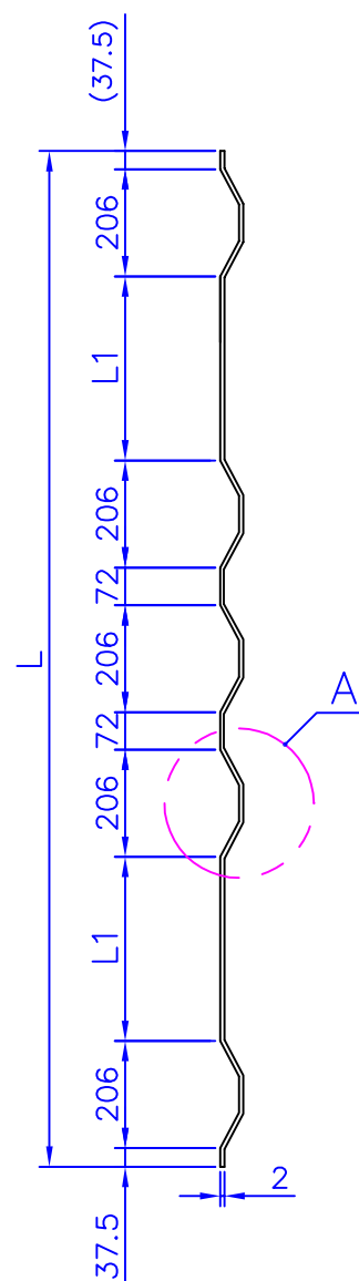
CIMC-D04-03A/B 五波门板
