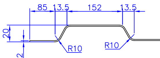
DETAIL C 2:1
