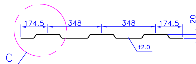
DETAIL B 2:1
