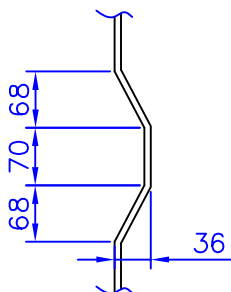
DETAIL A 2:1
