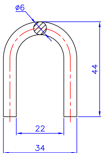
CIMC-D30-06 Ø6X44
