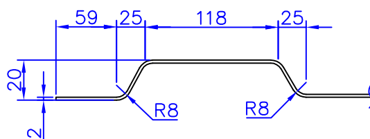
DETAIL C 2:1
